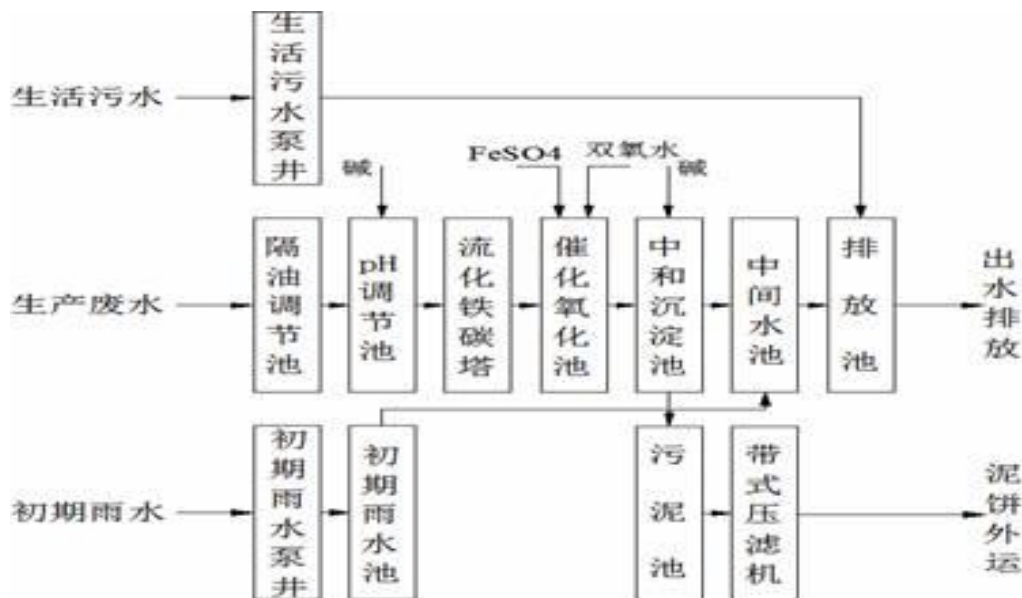
图 1 原有装置工艺流程简图
